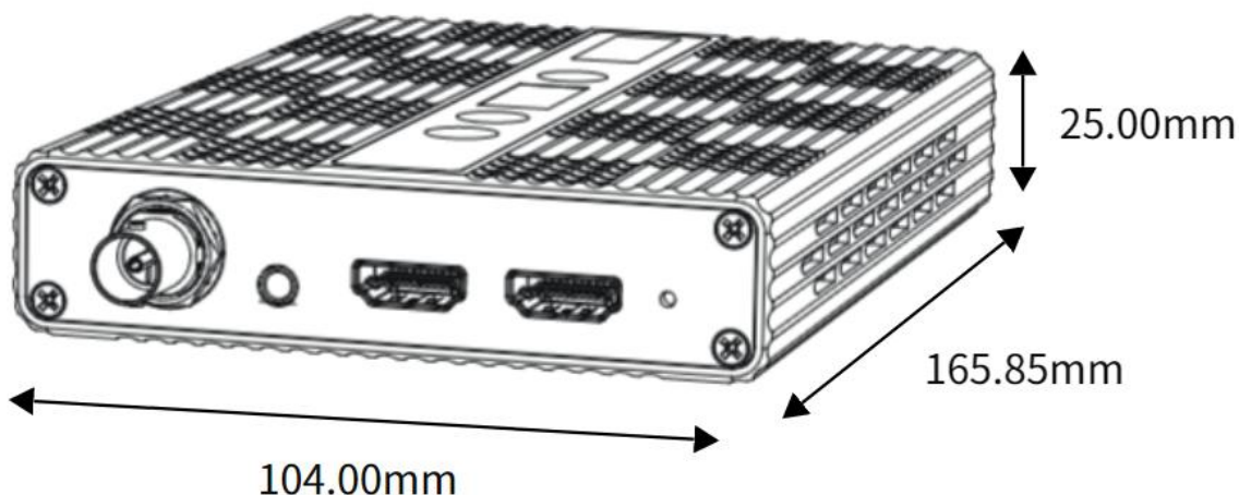
D350 产品尺寸图
