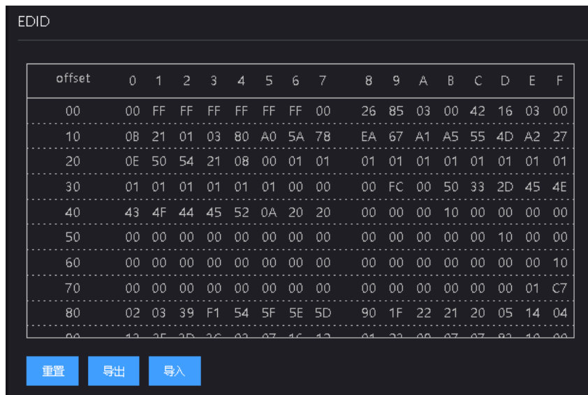
图 55 设置-EDID 设置
